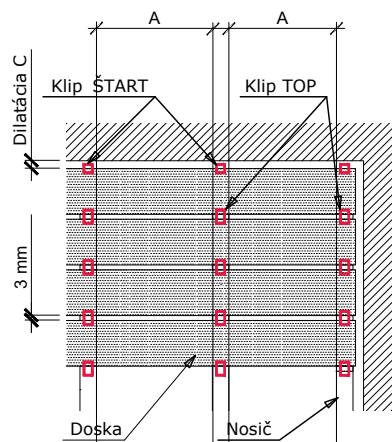
Obr. 4 Dilatačné medzery medzi doskami a medzi doskami a pevnou stenou.
