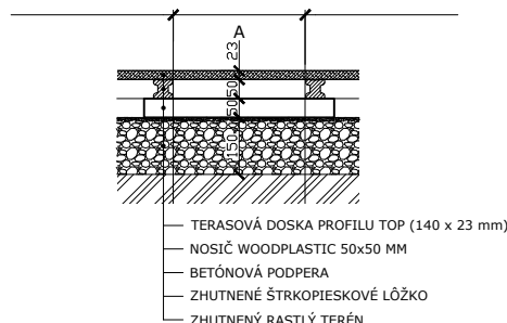
Obr. 1 Skladba terasy vrátane výšok pri použití nosičov WoodPlastic® 50 x 50 mm
