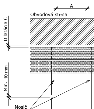
Obr. 2 Pokládka nosičov a vzdialenosti medzi nimi.
