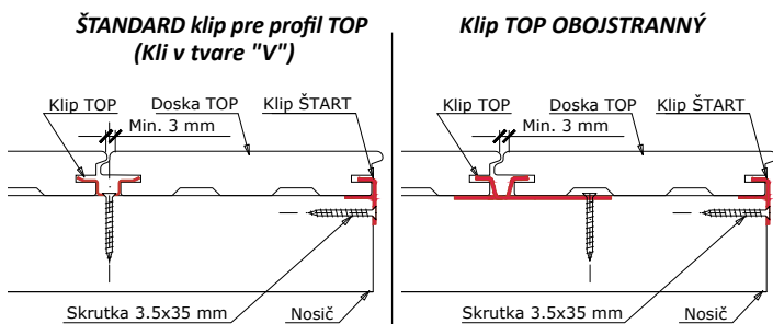
Obr. 3 Kotvenie terasových dosiek TOP pomocou nerezových klipov a skrutiek
