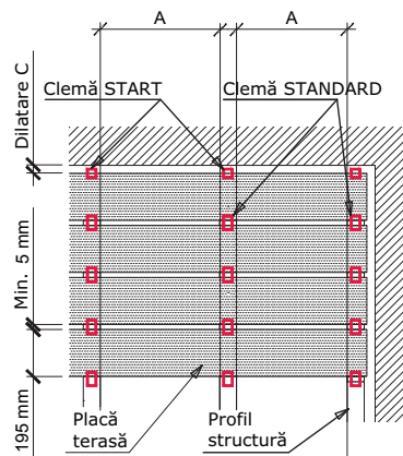
Fig. 4 - Instalarea plăcilor de terasă.
