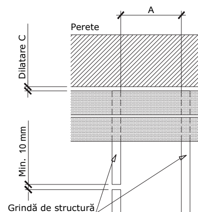
Fig. 2 - Instalarea grinzilor de structură și distanțele dintre ele.
