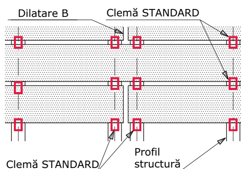
Fig. 5 - Conectarea capetelor plăcilor cu clemă STANDARD.
