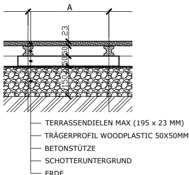
Abb.1 Terrassenaufbau inkl.Höhen durch en insatz Träger Woodplastic®
